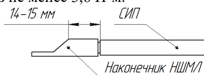
Рисунок 3.1 – СИП с наконечником НШМЛ
