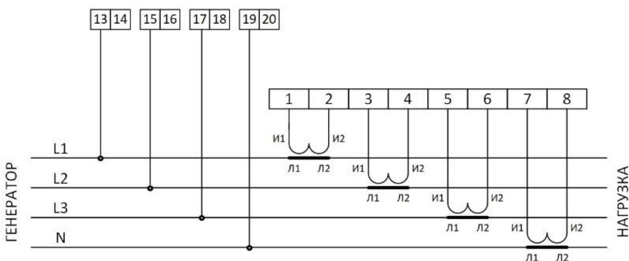
Рисунок Б.2 - Схема подключения через трансформаторы тока счетчиков полукосвенного включения в исполнении D и W
