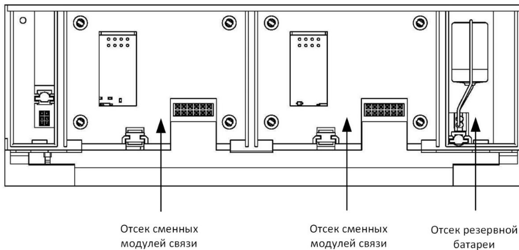
Рисунок А.5 - Счетчик в исполнении D с полукошвенного включения с снятой верхней крышкой и снятыми крышками отсеков
