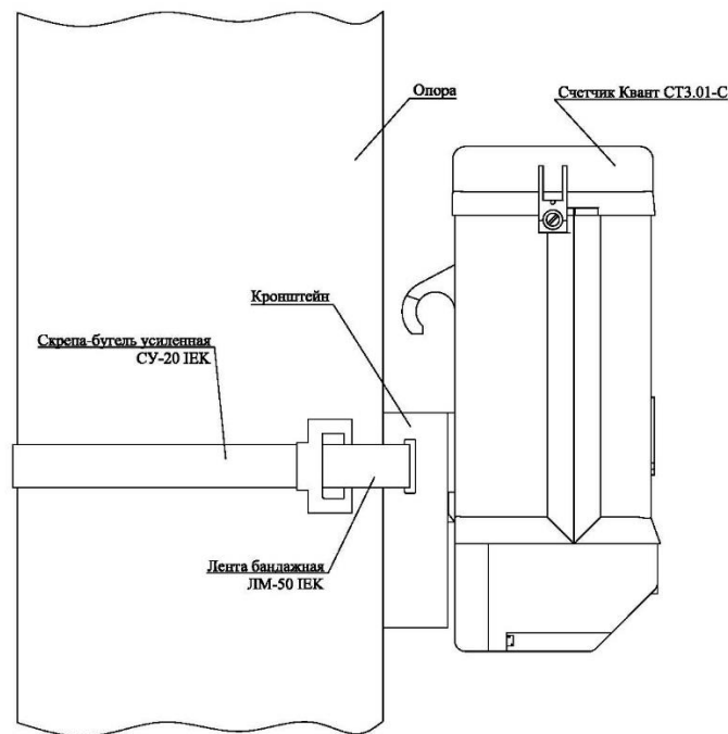
Рисунок 3.2 – Счетчик с кронштейном на опоре
