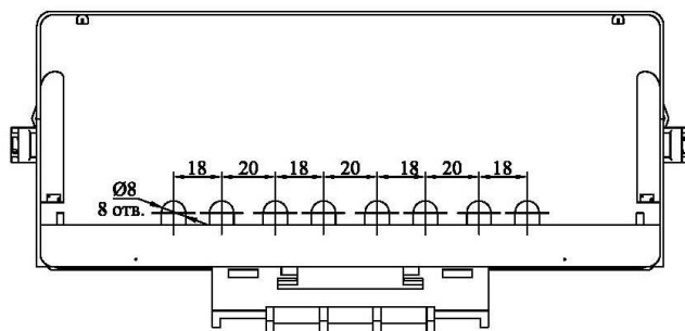
Рисунок А.6 - Размеры счетчика в исполнении С
