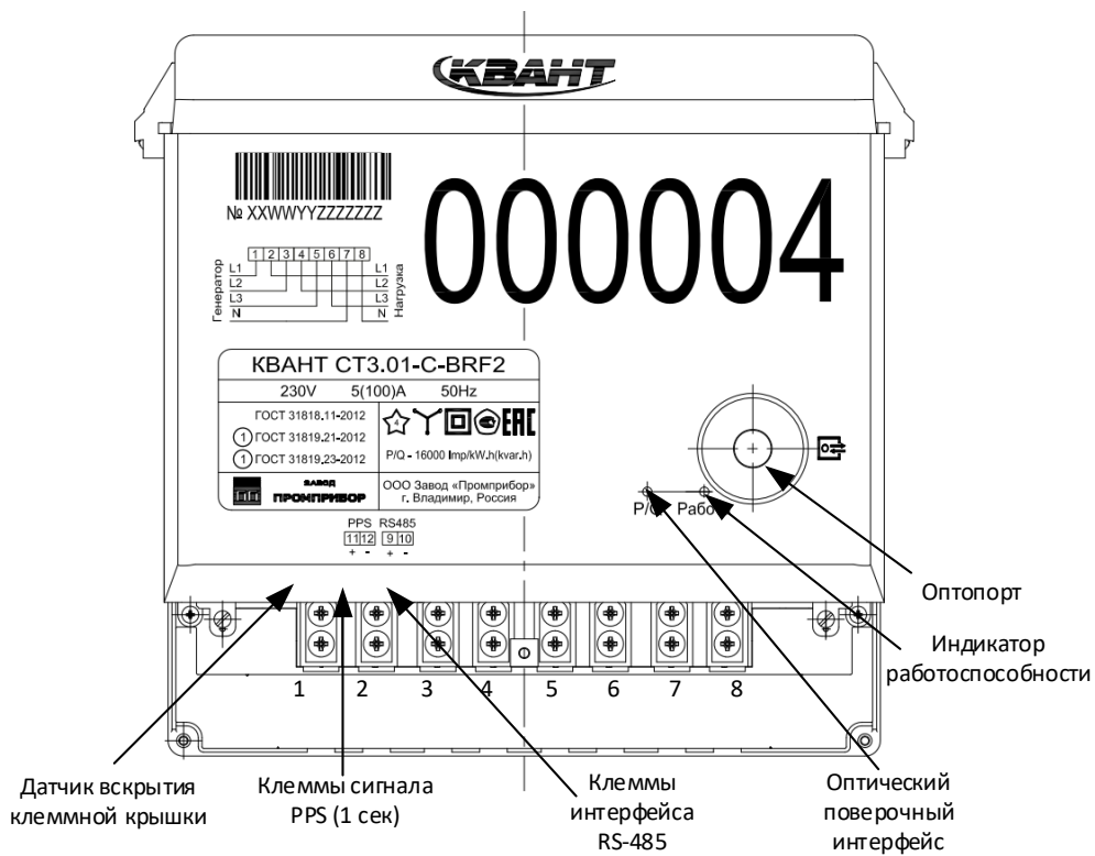
Рисунок А.7 - Счетчик в исполнении С со снятой клеммной крышкой
